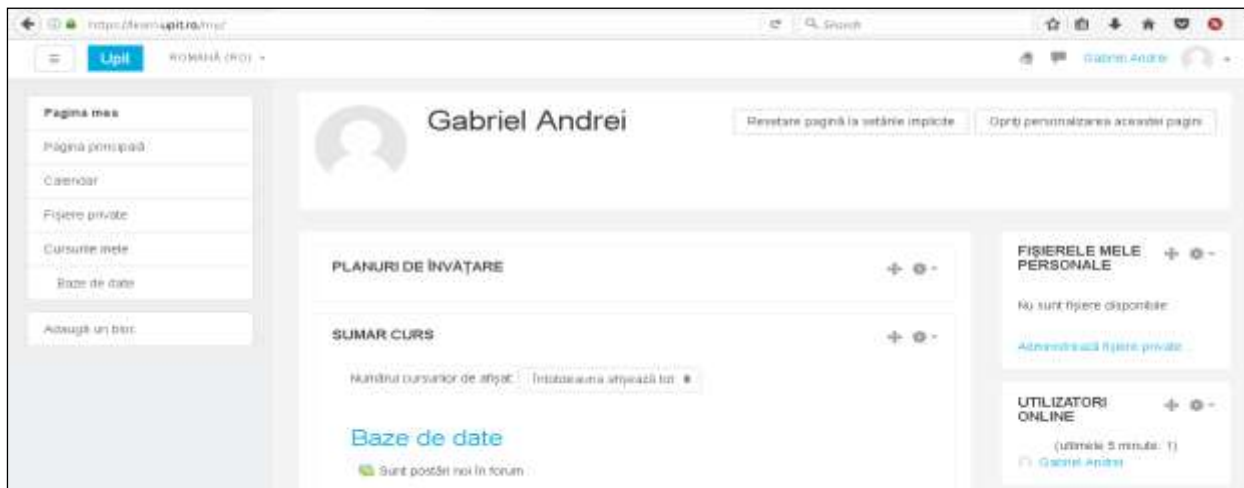
Fig. 4. Pagina principală
