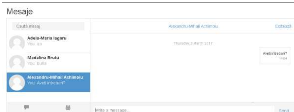
Fig. 10. Trimiterea mesajelor
